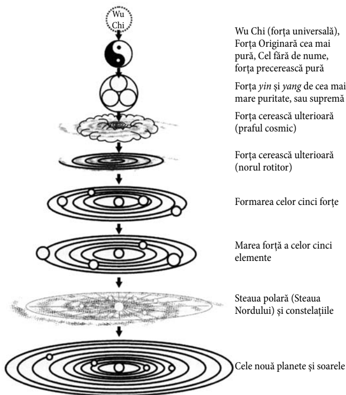
Fig. I.1. Formarea și evoluția universului
